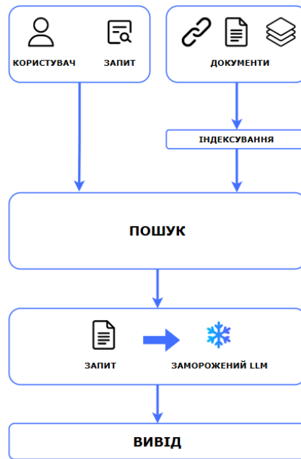
Рис. 1. Діаграма, що ілюструє типовий робочий процес RAG [4]
