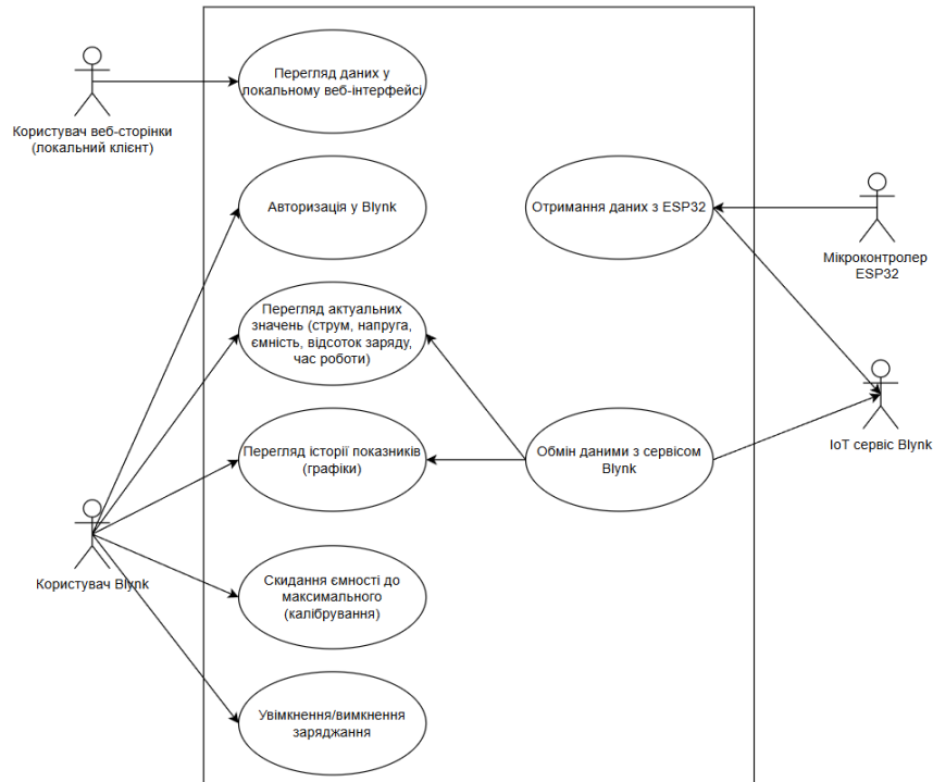
Рис. 1. Діаграма варіантів використання додатку
