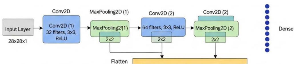
Рис. 1. Базова модель CNN
