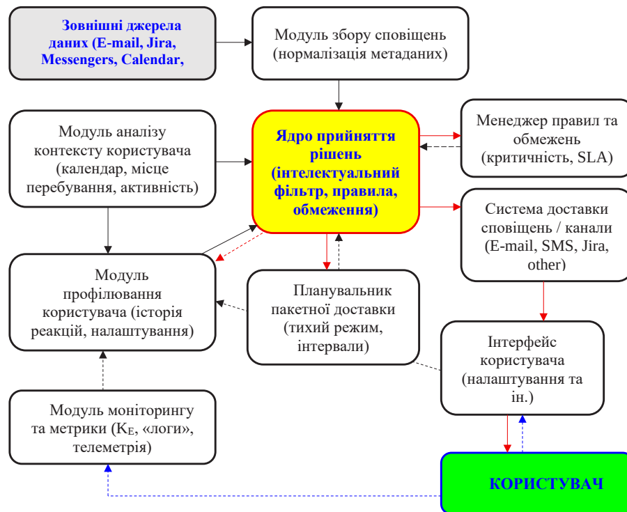
Рис. 1. Концептуальна модель інтелектуальної інформаційної системи, призначена для мінімізації негативного впливу цифрових сповіщень на продуктивність ІТ-фахівців
