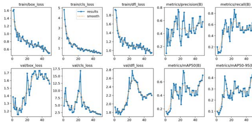
Рис. 4. Результати навчання моделі YOLOv8 для розпізнавання двох типів біоестиматорів активного мулу: криві втрат (train/val loss) та динаміка метрик точності (precision), повноти (recall) і середньої точності (mAP)
