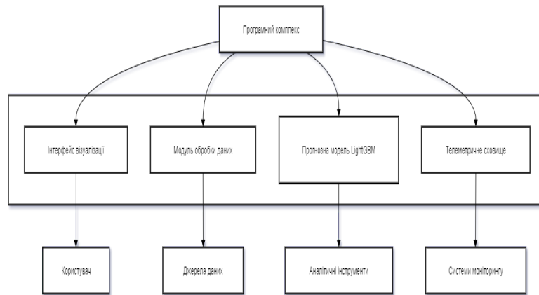
Рис. 1. Архітектура програмного комплексу прогнозування (ПКП)
