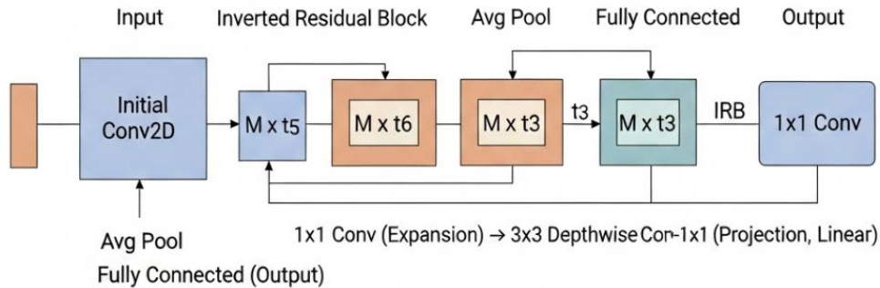
Рис. 4. Основні компоненти MobileNetV2
