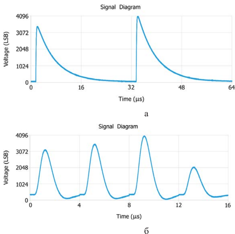
Рис. 1. Візуалізація оцифрованих спектрометричних сигналів з імпульсами різної форми: а – імпульси записані безпосередньо з детектора; б – імпульси отримані після попередньої обробки аналоговим фільтром Батерворта
