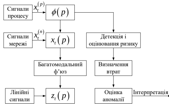
Рис. 1. Структурна схема пропонованої гібридної архітектури нейромережевої моделі
