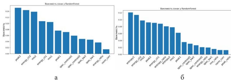
Рис. 3. Оцінка важливості ознак RandomForest для вектора: а) базового; б) повного
