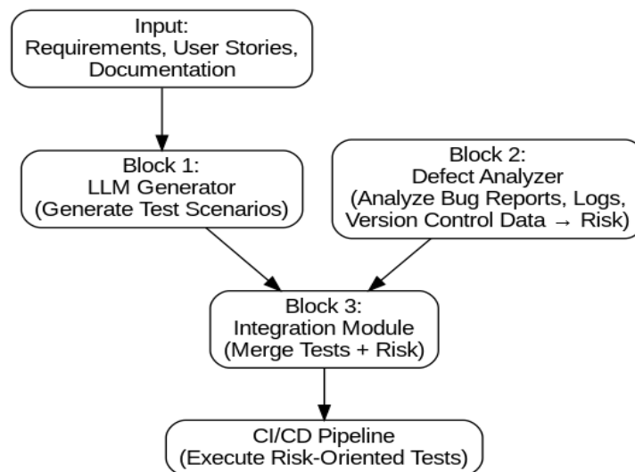
Рис. 1. Архітектурна модель гібридної системи генерації тестових сценаріїв
