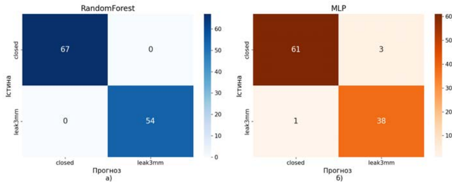
Рис. 4. Матриці плутанини на тестовому наборі для: а) RandomForest; б) MLP
