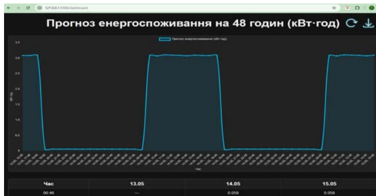
Рис. 4. Інтерфейс системи
