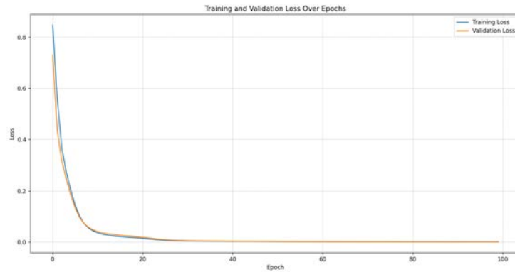
Рис. 2. Зміни значення функції втрат під час навчання моделі автоенкодера для формування представлення про крок сценарію
