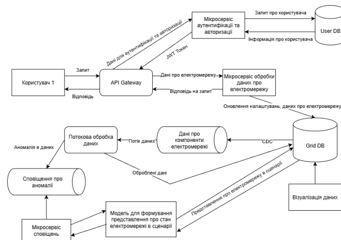
Рис. 7. Архітектура програмного забезпечення
