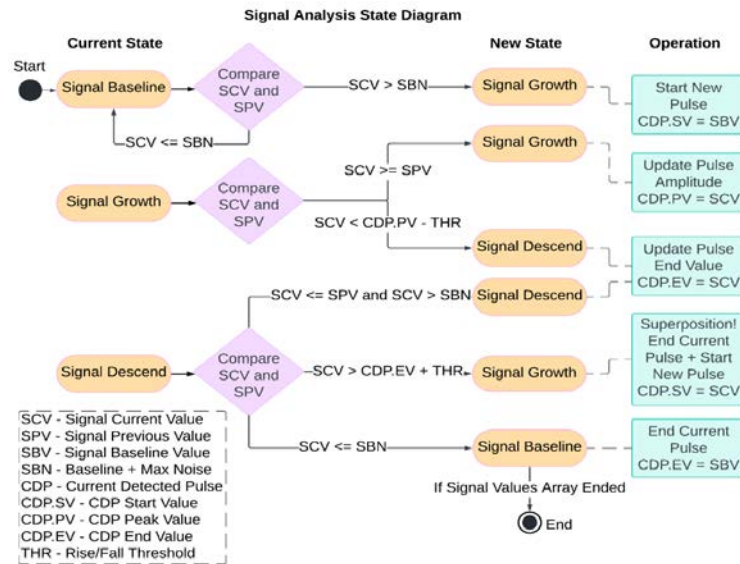
Рис. 3. UML діаграма станів, переходів між ними та пов'язаних з цим операцій в процесі аналізу відфільтрованого сигналу розробленим методом
