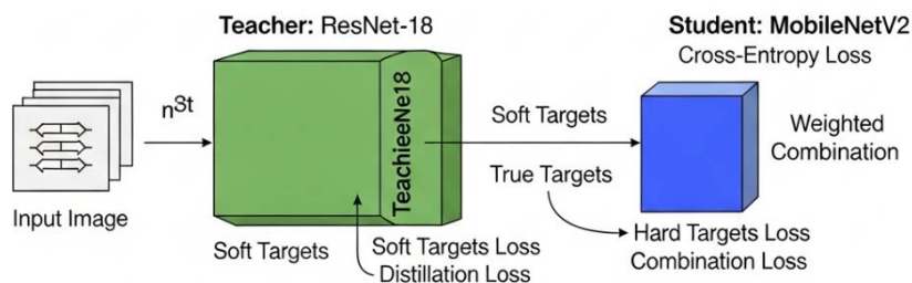
Рис. 3. процес Knowledge Distillation
