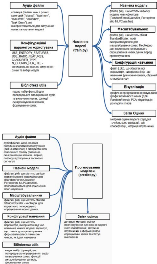
Рис. 1. Контекстна діаграма процедури: а) навчання моделей; б) тестування
