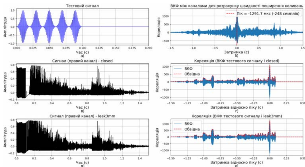
Рис. 2. Часовий та кореляційний аналіз діагностичних сигналів: а) тестовий сигнал; б) ВКФ каналів; в) сигнал правого каналу за відсутності витоку; г) ВКФ для стану закрито; д) сигнал правого каналу за наявності витоку 3 мм; е) ВКФ для стану з витоком 3 мм
