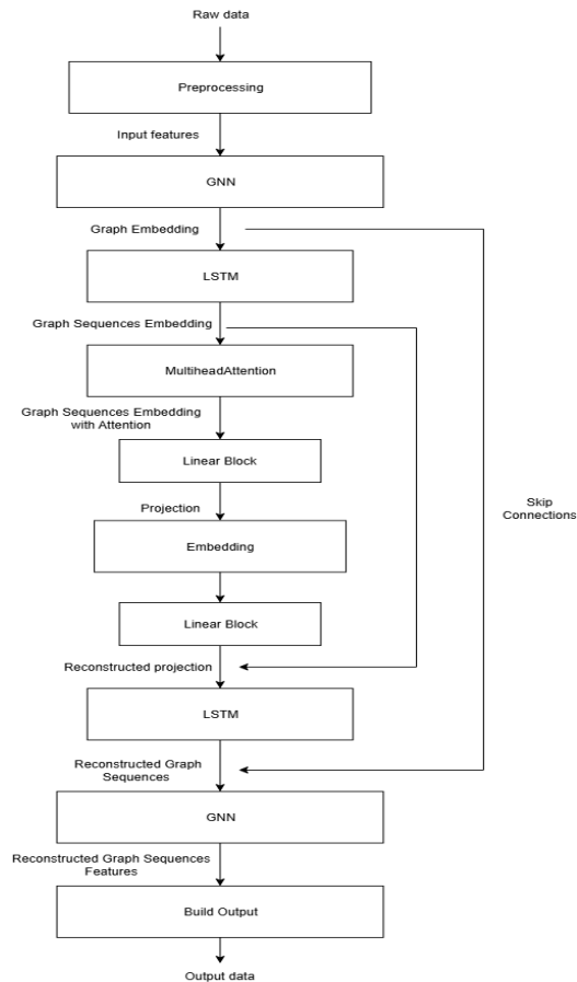
Рис. 4. Структура автоенкодера для формування представлення про послідовність кроків сценарію
