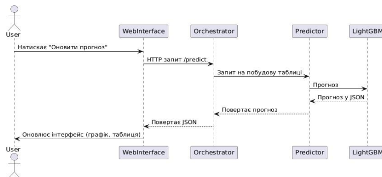
Рис. 5. Діаграма послідовності оновлення прогнозу енергоспоживання
