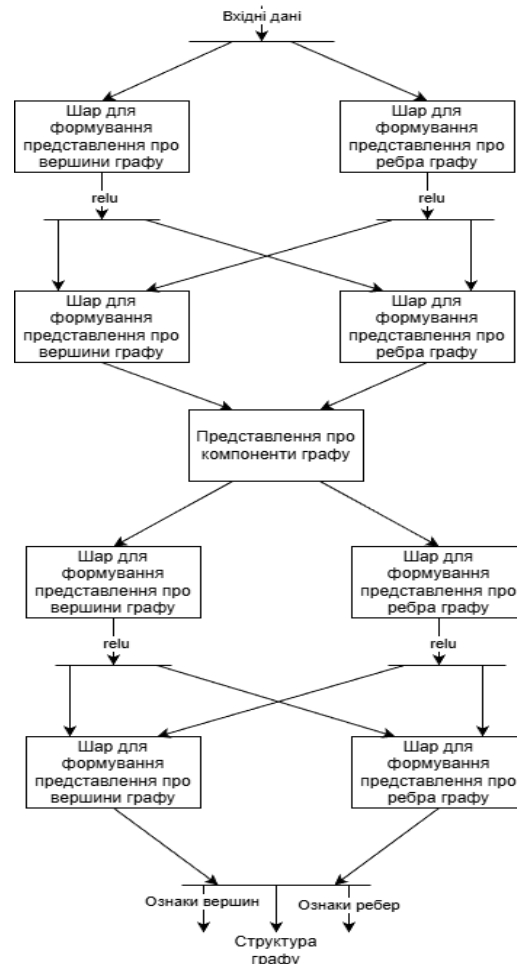
Рис. 1. Структура автоенкодера для формування представлення про вершини та ребра електромережі в кроці сценарію
