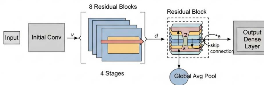
Рис. 2. ResNet-18
