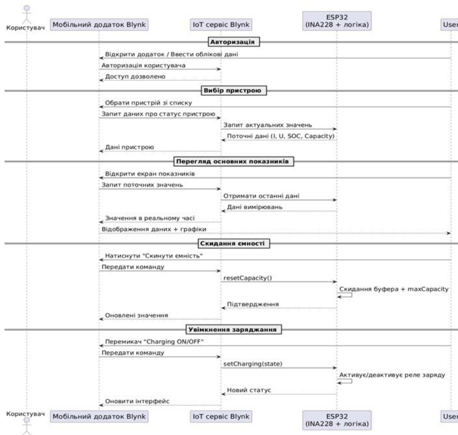
Рис. 2. Діаграма послідовності
