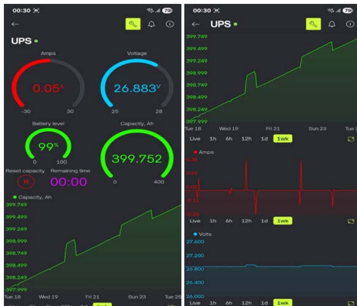
Рис. 5. Головний екран
