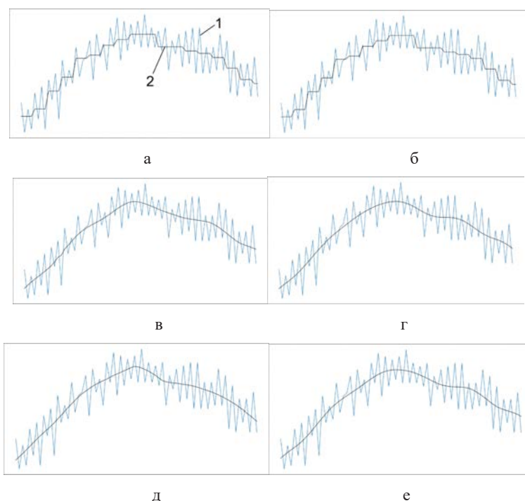
Рис. 2. Вигляд відфільтрованого сигналу (1 – оригінальний сигнал; 2 – відфільтрований сигнал) за допомогою дискретних вейвлет-перетворень при використанні різних материнських вейвлетів: а – Haar, б – db1, в – Bior6.8, г – db10, д – symlet4, е – symlet8
